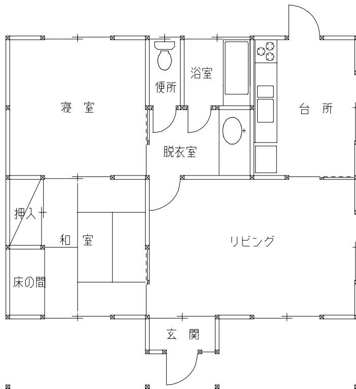
1階平面図 1/100
